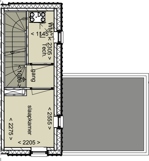
2e verdieping
