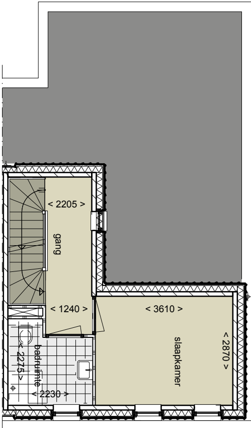
1e verdieping
